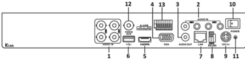
4 路 TVI Hybrid 監控錄影機後背板圖
