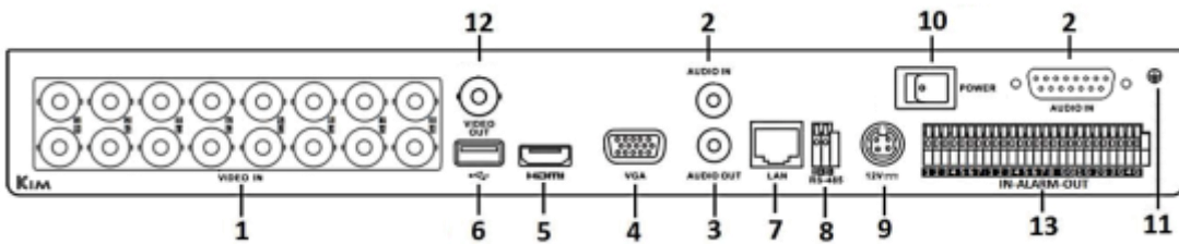
16 路 TVI Hybrid 監控錄影機後背板圖
