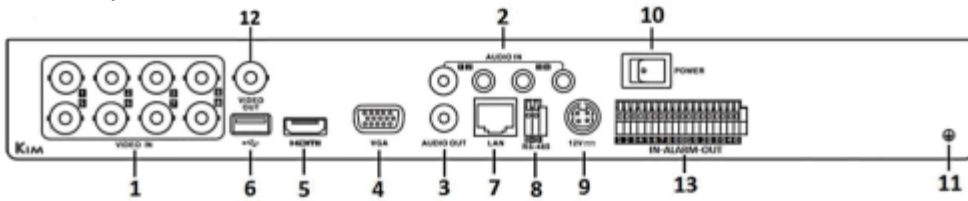
8 路 TVI Hybrid 監控錄影機後背板圖
