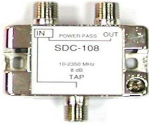
SDC-108 衛星一分歧器
