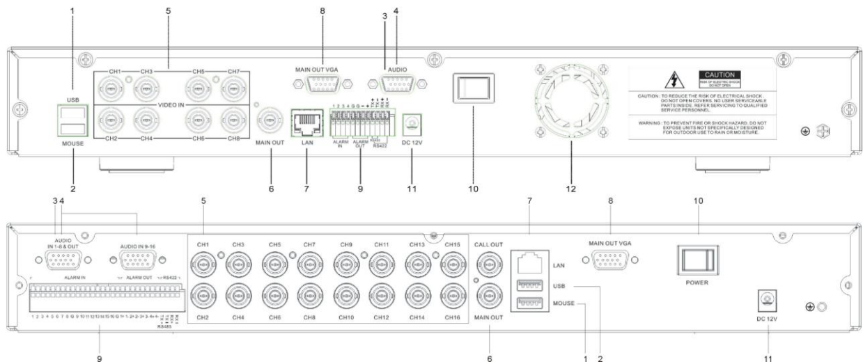
(8-16CH_DVR 後背板圖示)
